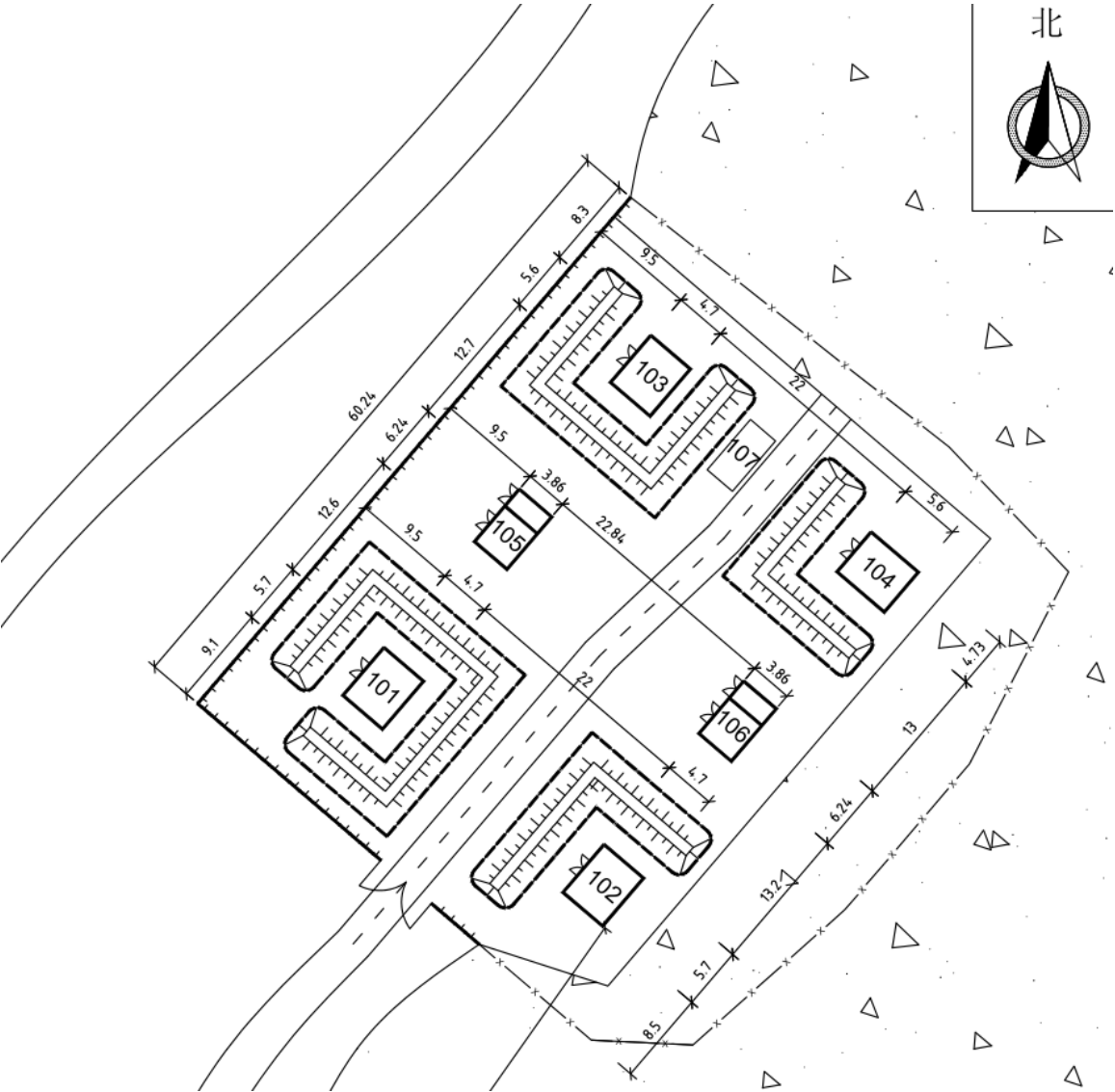
图 2-1 库区平面布置图
